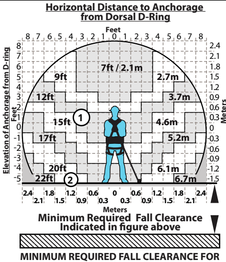
Figure 12 - Dégagement de chute minimum requis pour le FT-X pour les utilisateurs de 59 à 141 k (130 à 310 lb)
