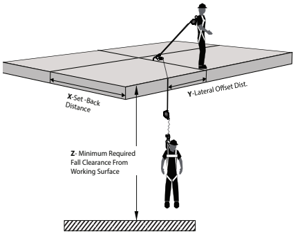
Figura 11 - Anclaje no suspendido de MRFC
