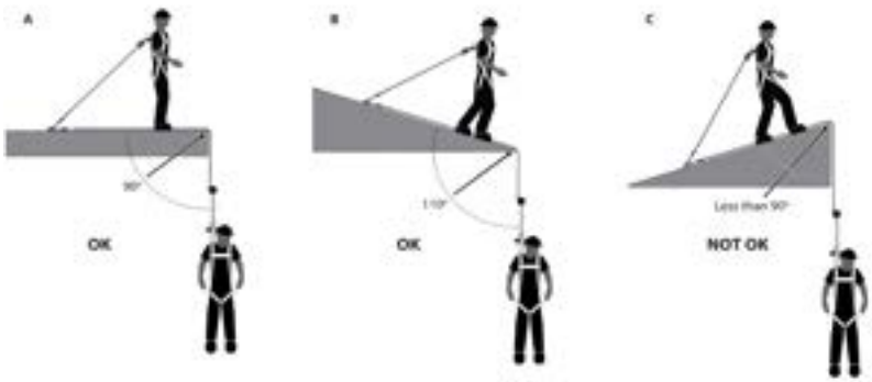
Figura 7: Redireccionar ángulo de borde delantero de cuerda de salvamento
