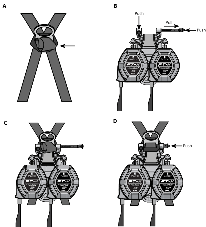
Figure 6 - Installation du bord d'attaque SRL-P de classe 2 FT-X EdgeCore
