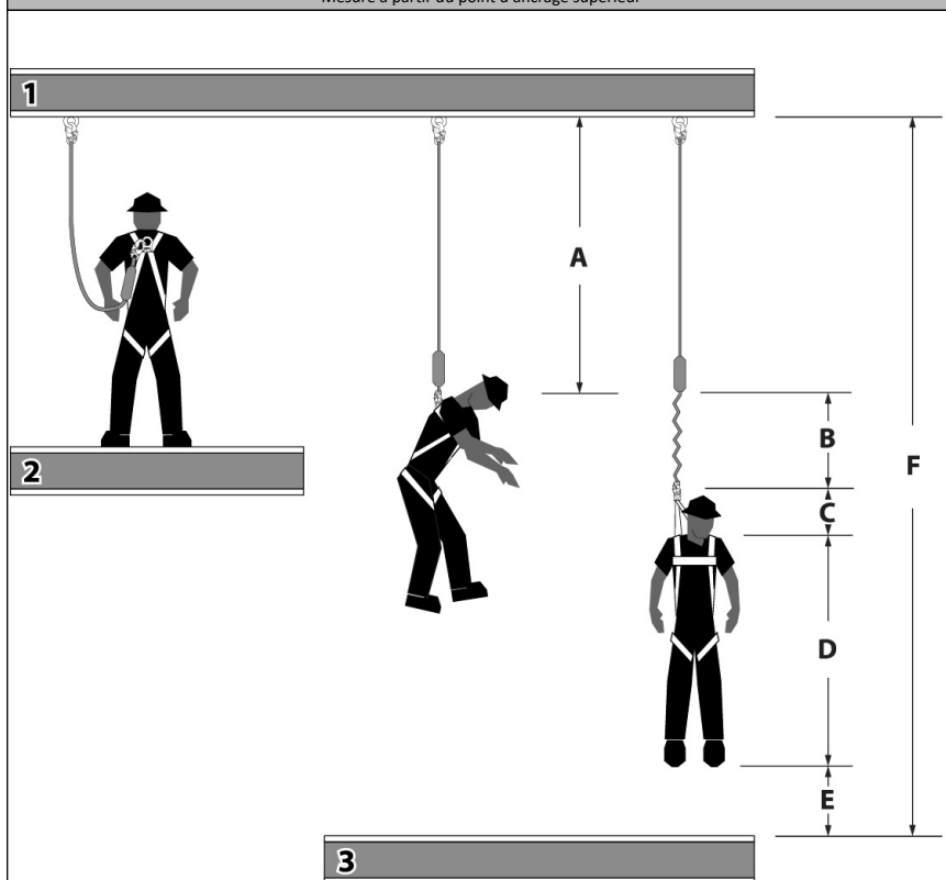
Figure 1 - Dégagement minimal requis en cas de chute : Cordon amortisseur d'énergie de 6 pieds. Mesuré à partir du point d'ancrage supérieur
